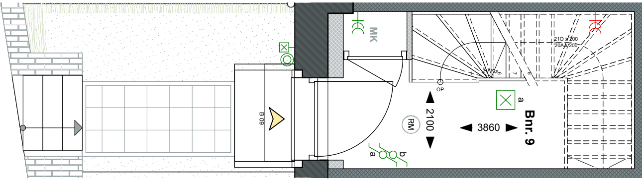
Begane grond - 1:50
