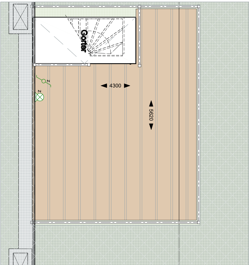
Dakterras - 1:50
