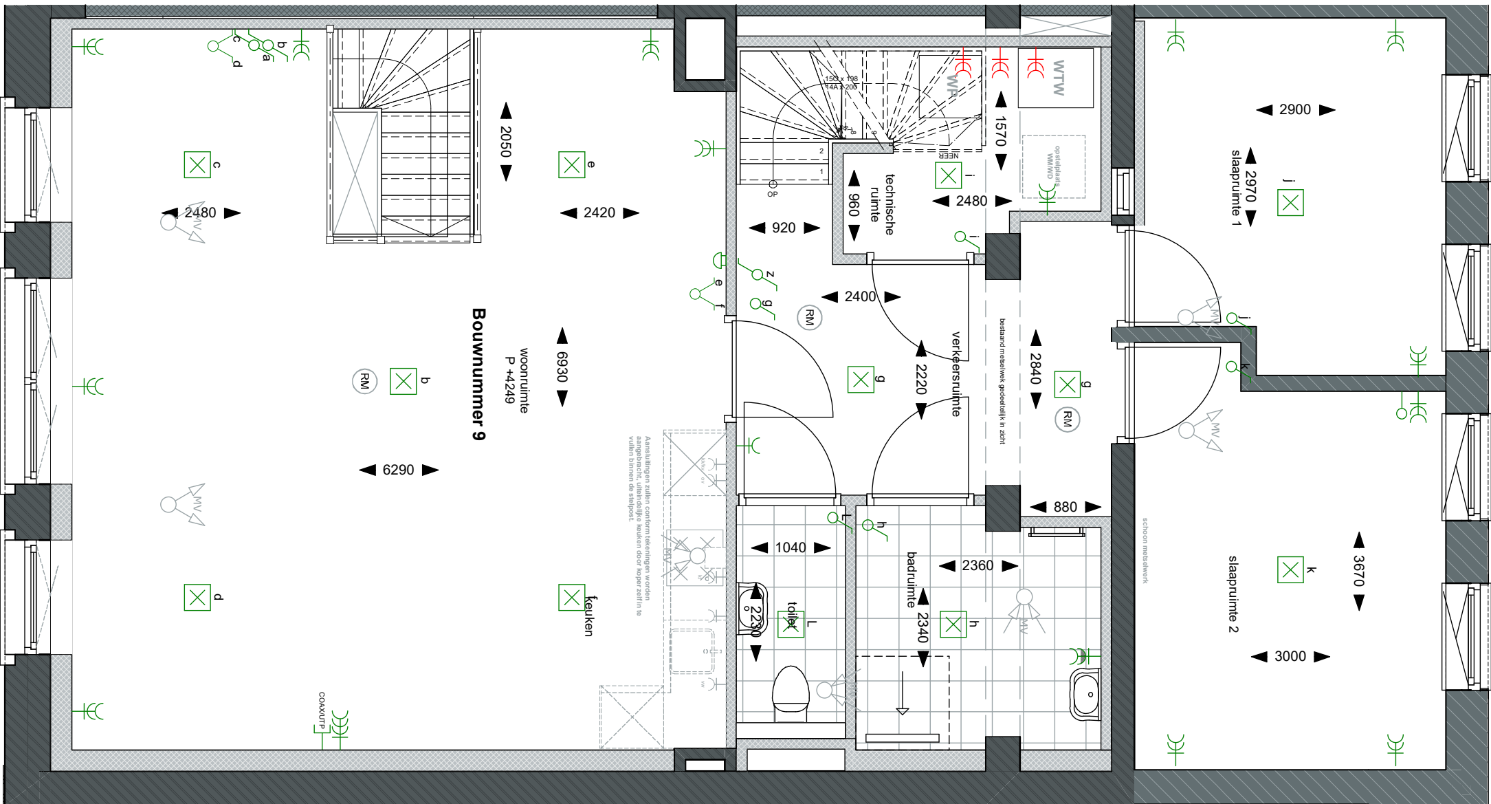
Eerste verdieping - 1:50
